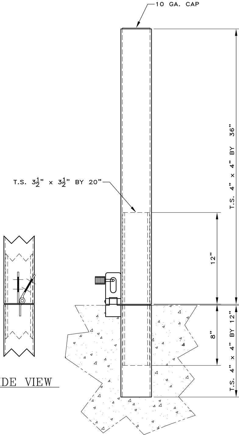
ELEVATION
