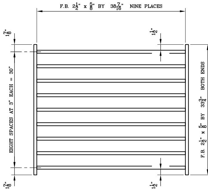
BAR GRATE
