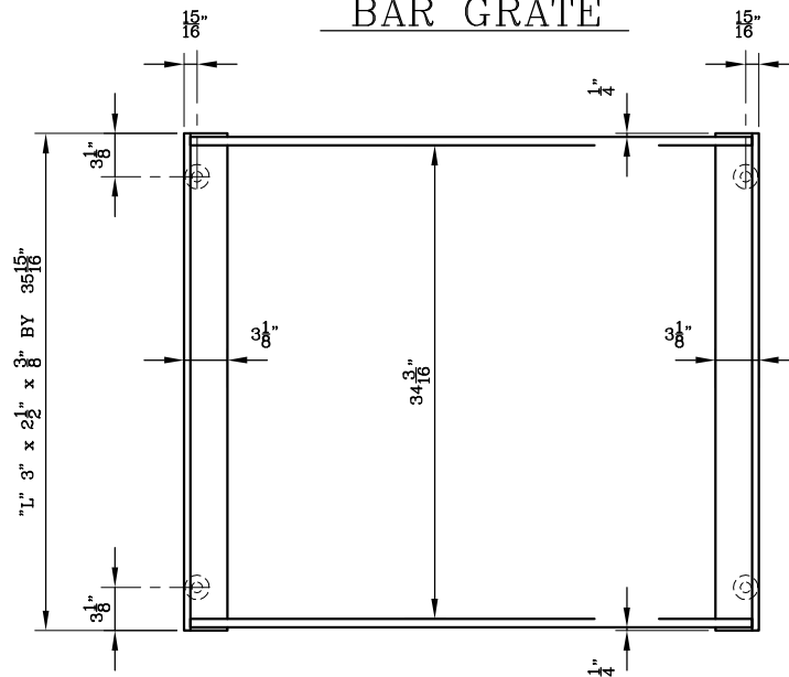
BAR GRATE
